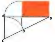
Золотий перетин Точка E, що позначає золотий поділ відрізка AB, знаходиться шльхом креслення дуги AD, потім дуги DE; у допоміжному трикутнику ABC: AC=AB/2; угорі – прямокутник із сторонами, які відповідають золотому перетину
